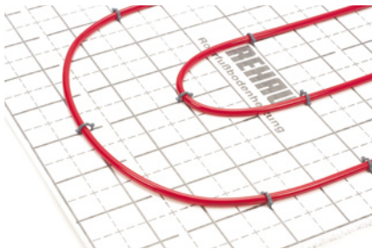
Pripínáčikový systém Tacker: úsporné systémové riešenie
