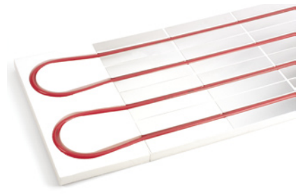
Podlahové vykurovanie v kompaktnom „suchom systéme“ s výškou 30 mm bez betonáže poteru, prekrytie sadrovláknitými doskami 25 mm
